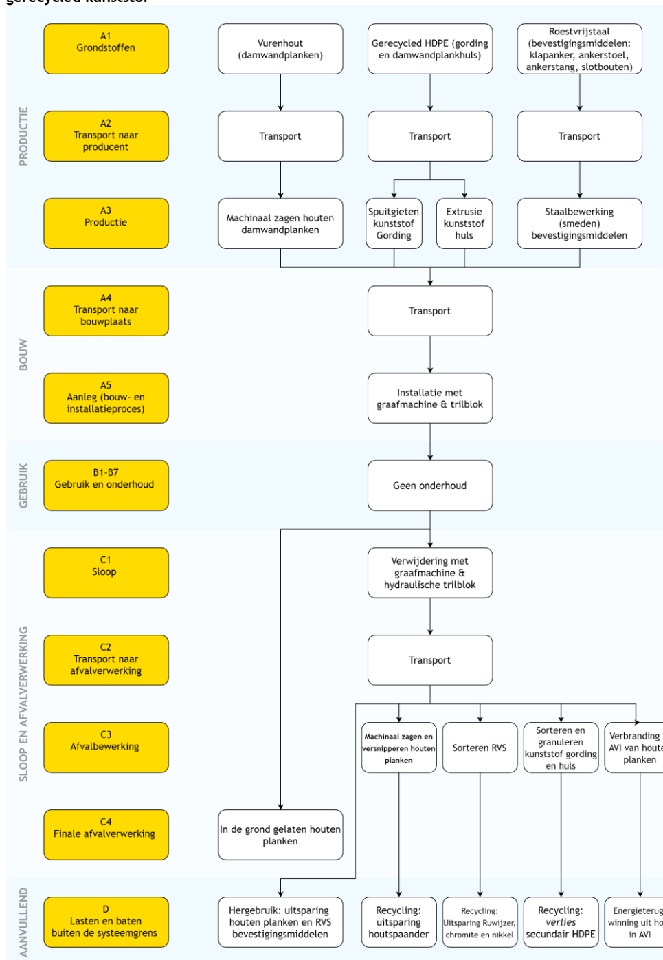
Figuur 1 - Levenscyclusfasen en belangrijkste processtappen van de damwand van Europees naaldhout en gerecycled kunststof
