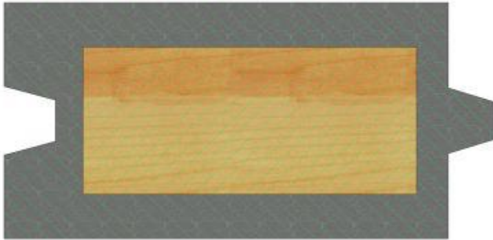
Figuur 3 - Doorsnede van damwandplank met huls
