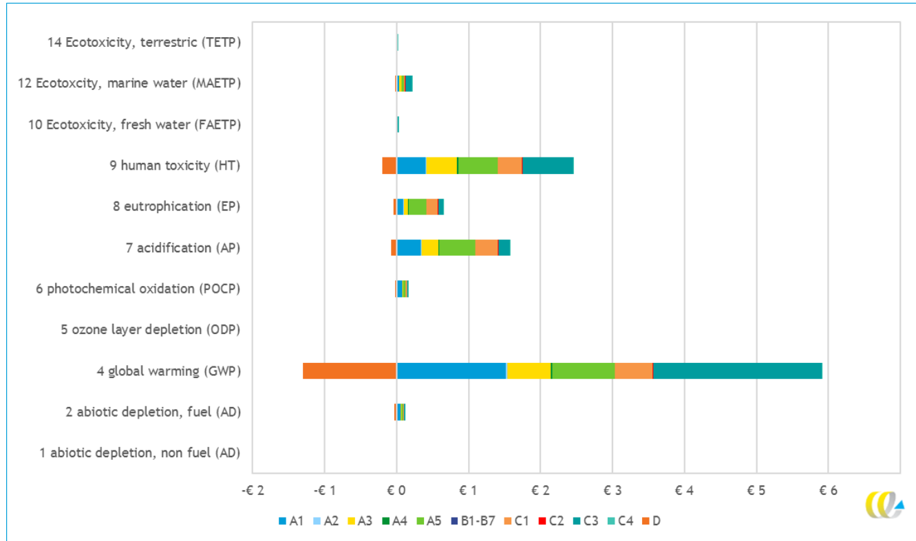
Figuur 4 - Gewogen milieuprofiel (MKI, in €) van één strekkende meter duiker van PVC, opgedeeld in levensfasen (exclusief 30% categorie-opslag)
