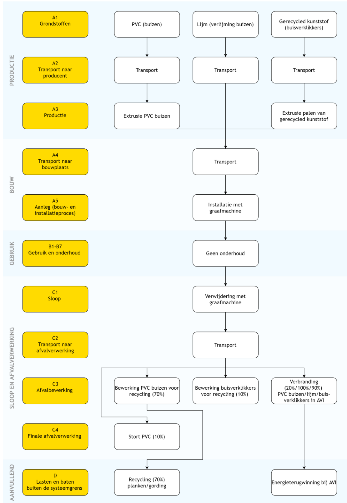
Figuur 1 - Levenscyclusfases en belangrijkste processtappen van een duiker van PVC
