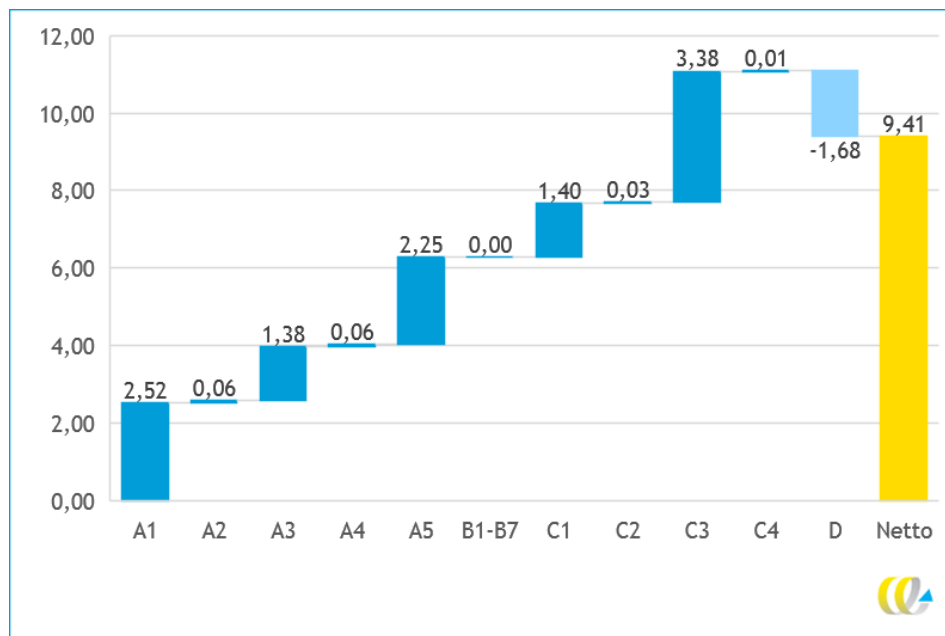
Figuur 3 - MKI-scores voor één strekkende meter duiker van PVC, opgedeeld in levensfasen (exclusief 30% categorie-opslag)
