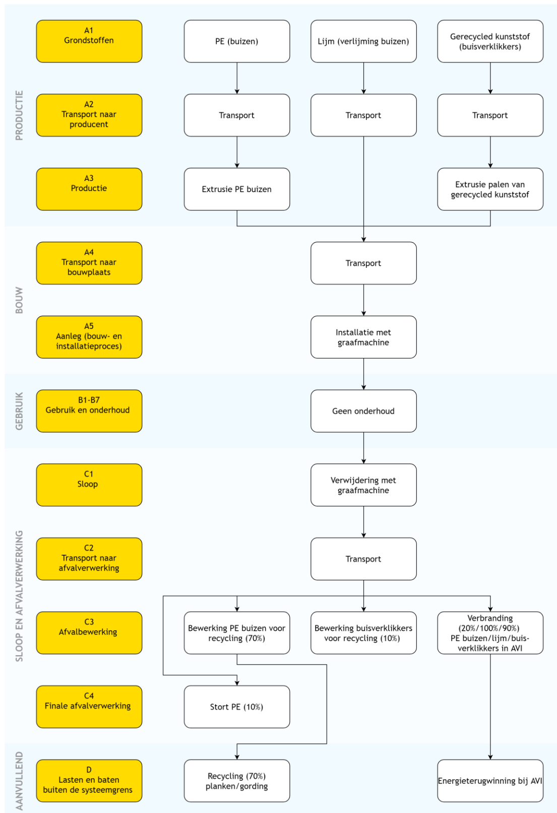
Figuur 1 - Levenscyclusfases en belangrijkste processtappen van een duiker van PE
