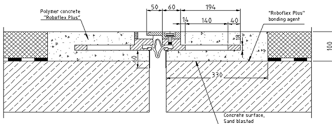
Onverankerde nosing joint van polymerebeton met stripverankering met sinusplaten (1.4a2)
