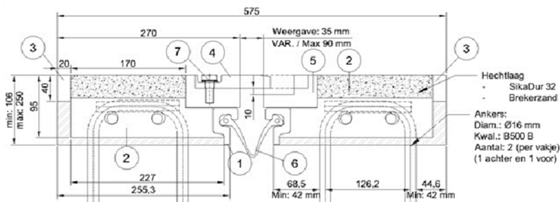
Figuur 2: Voegovergang 1.2b2, technische tekening type BR-Silent
