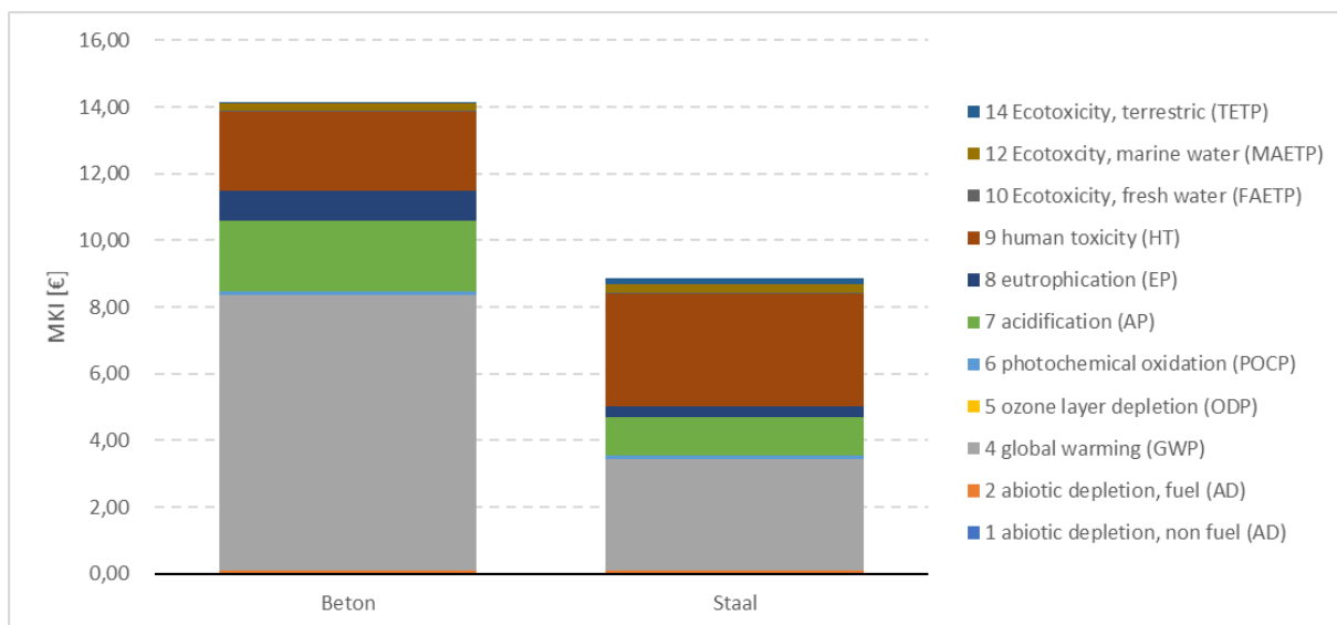
Figuur 3 Zwaartepunt A1-A3 Doorgaand Gewapend Beton C30/37 CEM III/B
