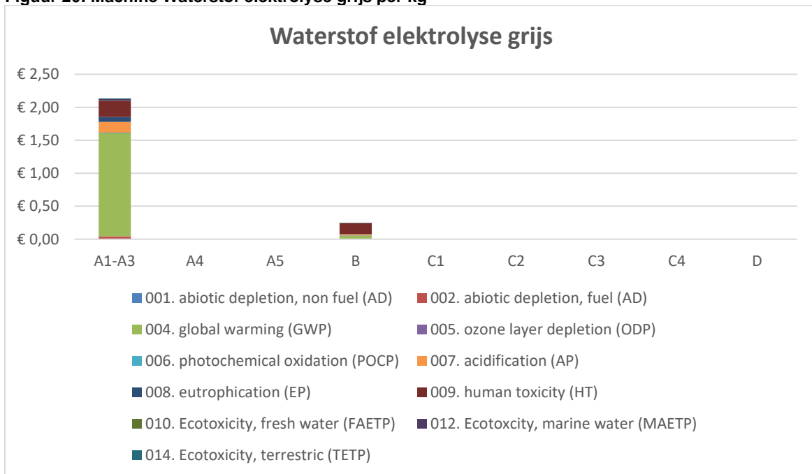
Figuur 20: Machine Waterstof elektrolyse grijs per kg
