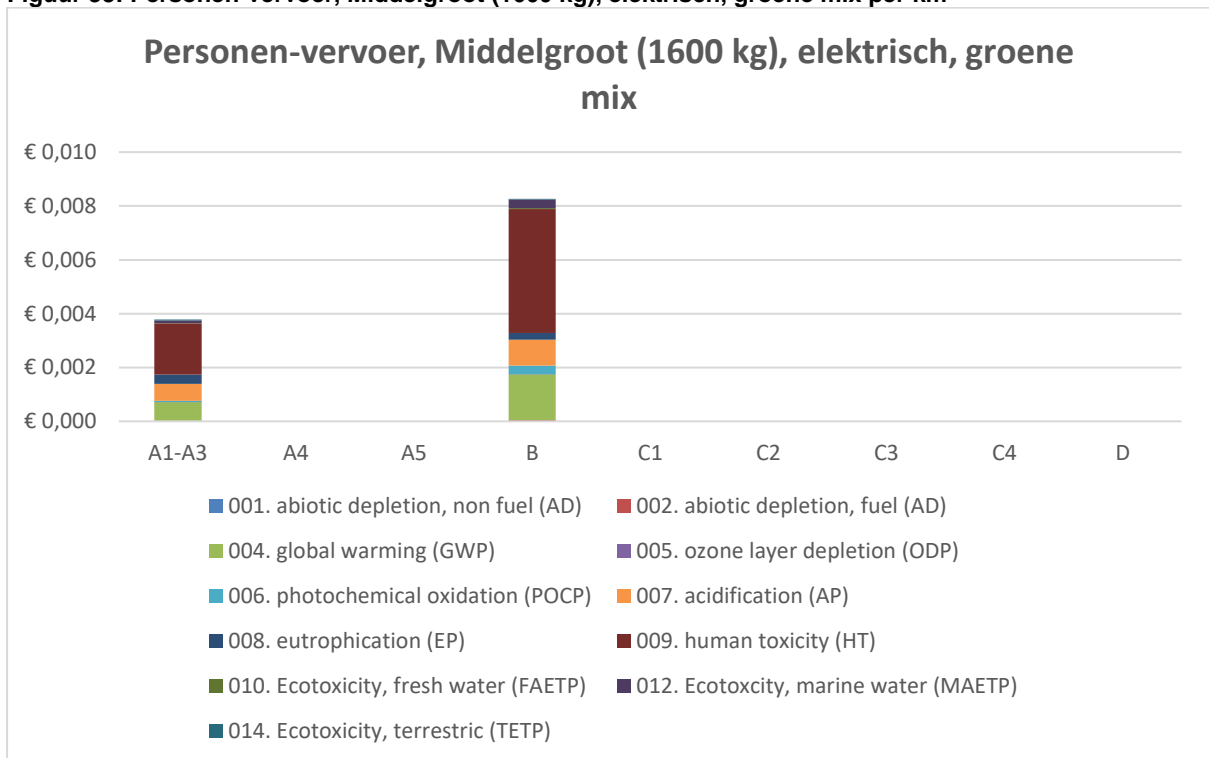
Figuur 33: Personen-vervoer, Middelgroot (1600 kg), elektrisch, groene mix per km
