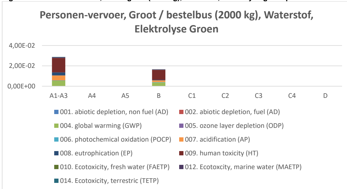
Figuur 45: Personenvervoer, Middelgroot (1600 kg), Waterstof, Elektrolyse groen per km
