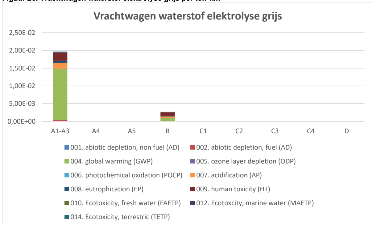
Figuur 26: Vrachtwagen waterstof elektrolyse grijs per ton*km
