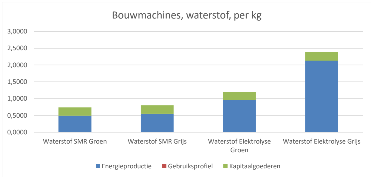
Figuur 5 Gewogen resultaten bouwmachines, waterstof, per kg
