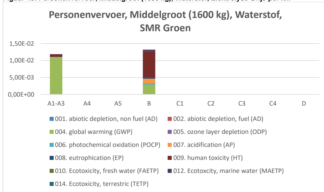
Figuur 43: Personenvervoer, Middelgroot (1600 kg), Waterstof, Elektrolyse Grijs per km
