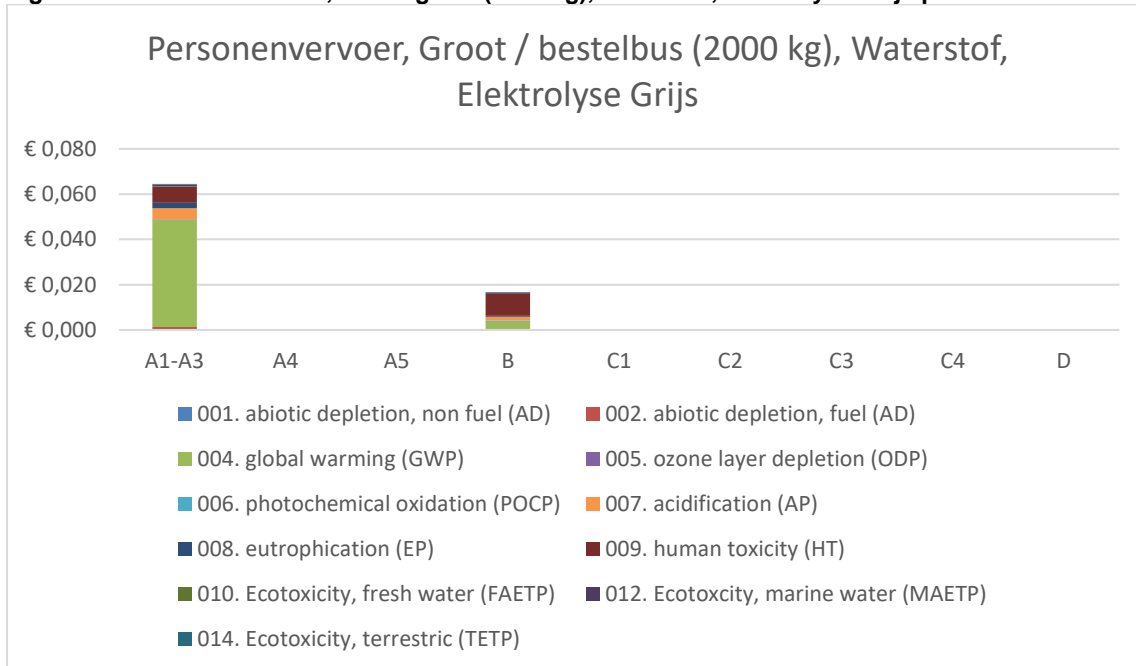
Figuur 44: Personenvervoer, Middelgroot (1600 kg), Waterstof, Elektrolyse Grijs per km
