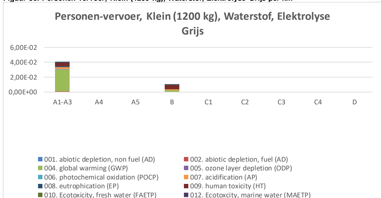
Figuur 36: Personen-voervoer, Klein (1200 kg), Waterstof, Elektrolyse Grijs per km
