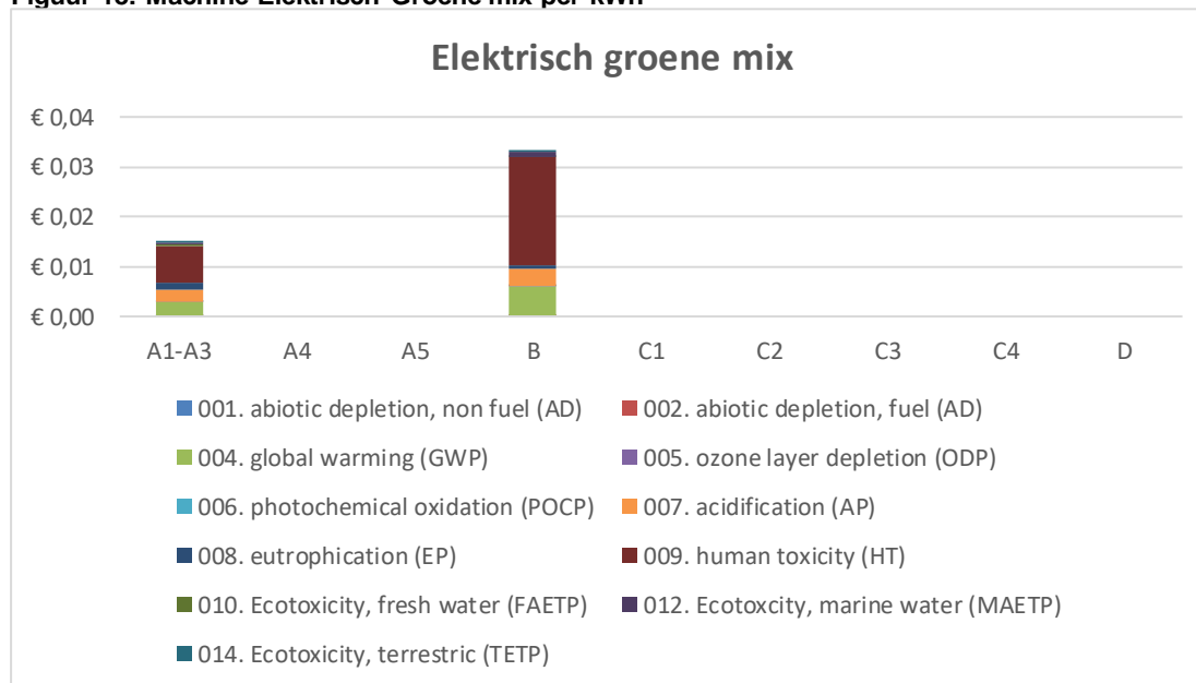
Figuur 18: Machine Elektrisch Groene mix per kWh
