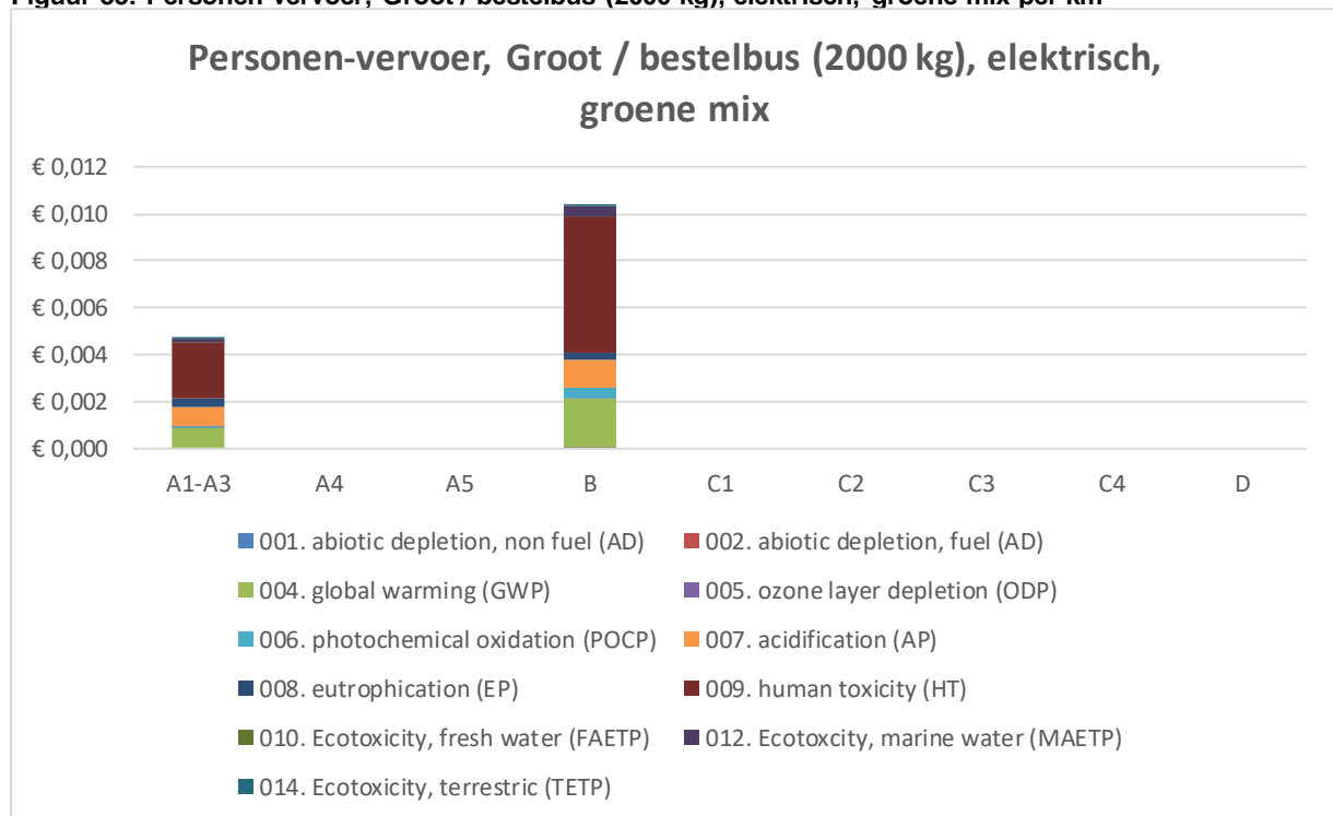
Figuur 35: Personen-voervoer, Groot / bestelbus (2000 kg), elektrisch, groene mix per km
