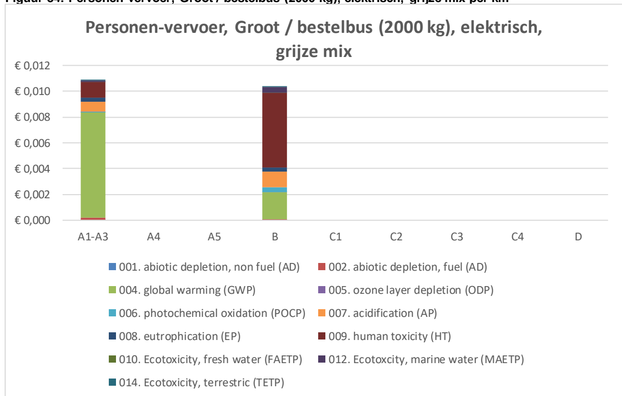
Figuur 34: Personen-voervoer, Groot / bestelbus (2000 kg), elektrisch, grijze mix per km
