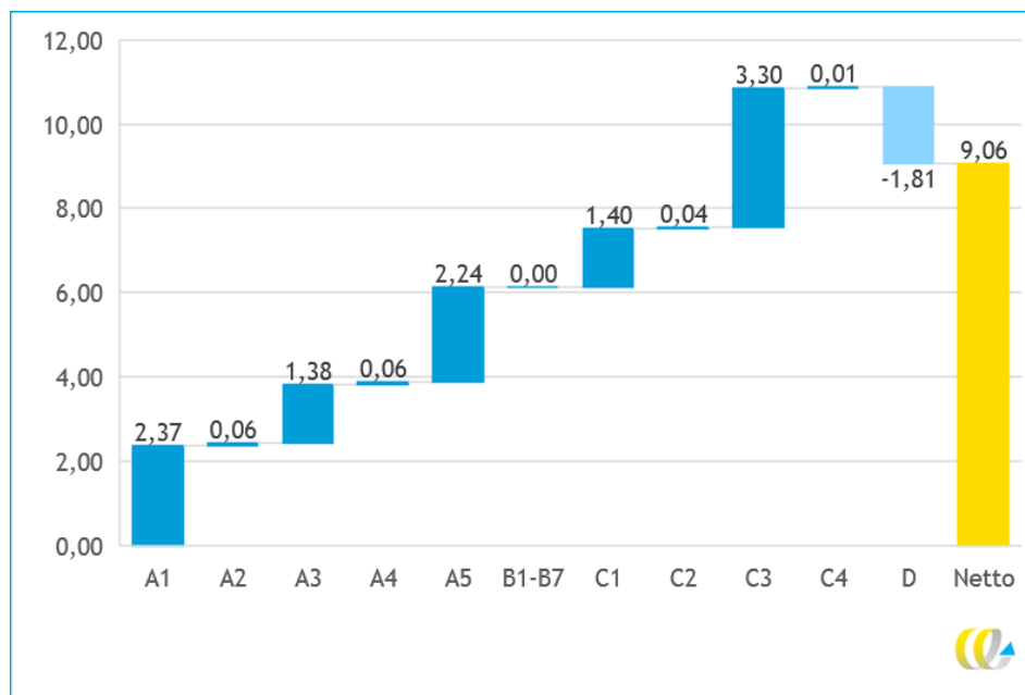
Figuur 3 - MKI-scores voor één strekkende meter duiker van PE, opgedeeld in levensfasen (exclusief 30% categorie-opslag)
