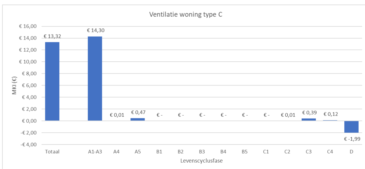
Figuur 1: Bijdrage aan MKI per module, ventilatie woning, type C, stuks
